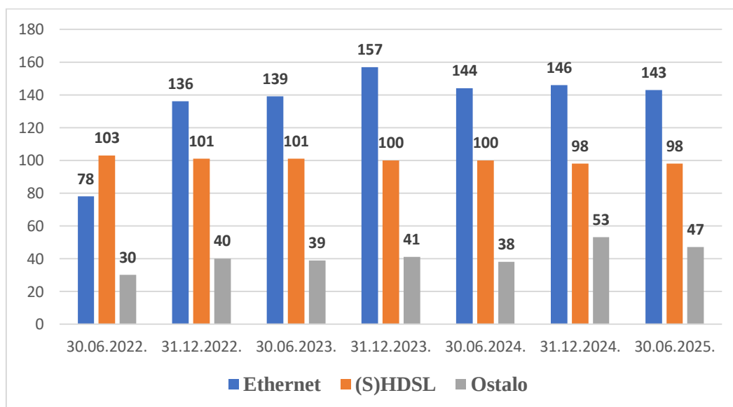
Grafikon 7: Ukupan broj priključnih tačaka na kojima se pružaju usluge garantovanih kapaciteta prema tehnologiji u analiziranom periodu
