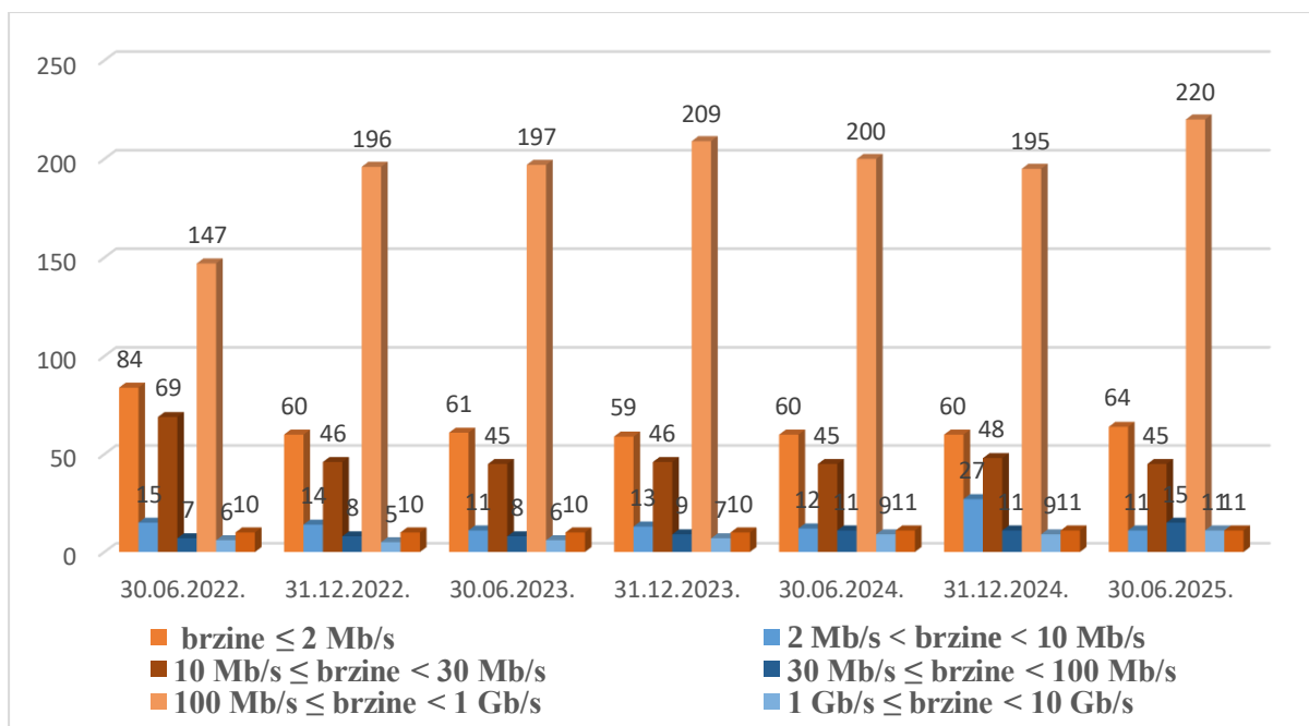
Grafikon 6: Ukupan broj priključnih tačaka na kojima se pružaju usluge garantovanih kapaciteta po kapacitetima na veleprodajnom nivou u analiziranom periodu
