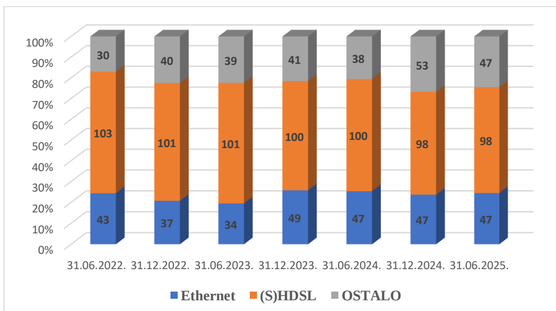
Grafikon 4: Broj korisnika usluga garantovanog kapaciteta operatora “Crnogorski Telekom” A.D. Podgorica prema tehnologiji
