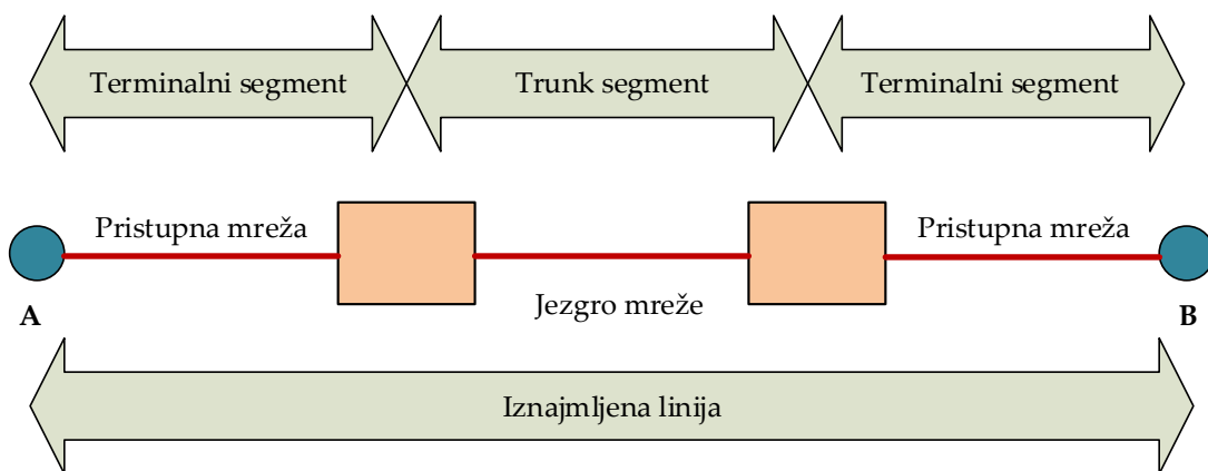
Slika 2: Šematski prikaz usluge garantovanog kapaciteta s kraja na kraj i usluge završnih segmenata garantovanih kapaciteta
